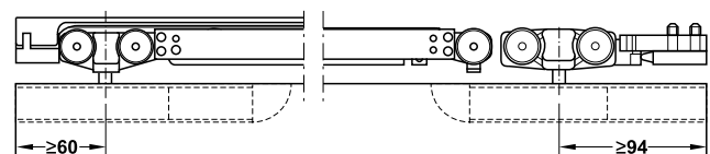
With soft and self closing mechanism on one side Giảm chấn và tự đóng một bên
