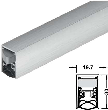
Retractable door seal DDS20 Thanh chắn bụi tự động DDS20
