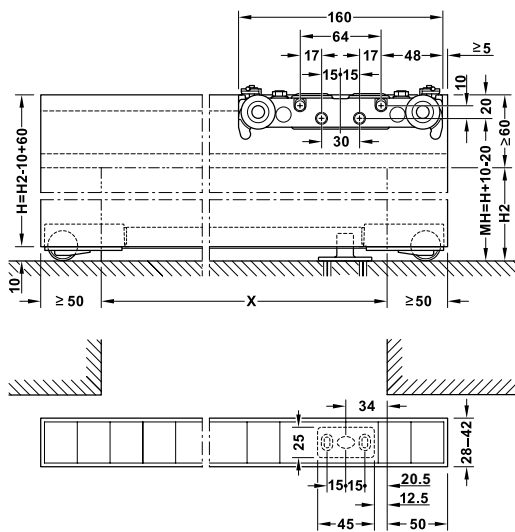
Floor guide on soft floor Dẫn hướng trên sàn mềm
