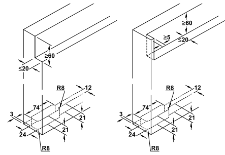
Panel preparation detail Chi tiết khoan cửa
