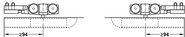
Without soft and self closing mechanism Không bao gồm cơ cấu giảm chấn
